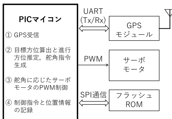
図 1 模擬人工衛星システムの構成
