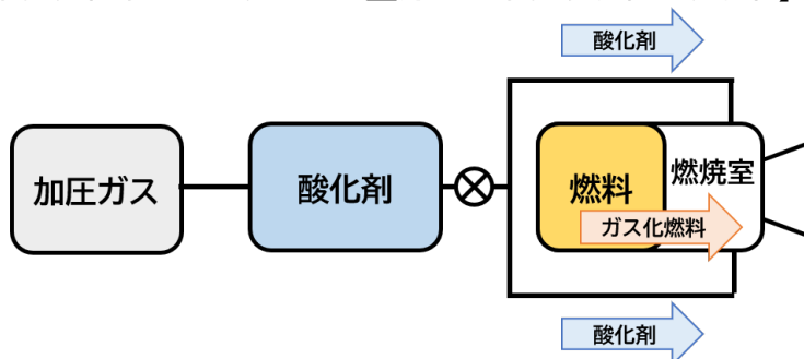
ガスハイブリッドロケットの模式図と TVC 装置
