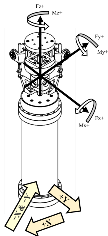
【TVC装置】
