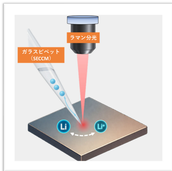
図 1 局所的な電気化学反応とラマン分光情報の同時計測が可能なオペランド顕微鏡の測定概念図。レーザーの焦点とガラスピペットの先端が一致しており、微小液滴を介して電気化学反応—本論文ではリチウムイオンの脱離・挿入プロセス—とラマン分光測定による構造変化の測定を可能としました。
